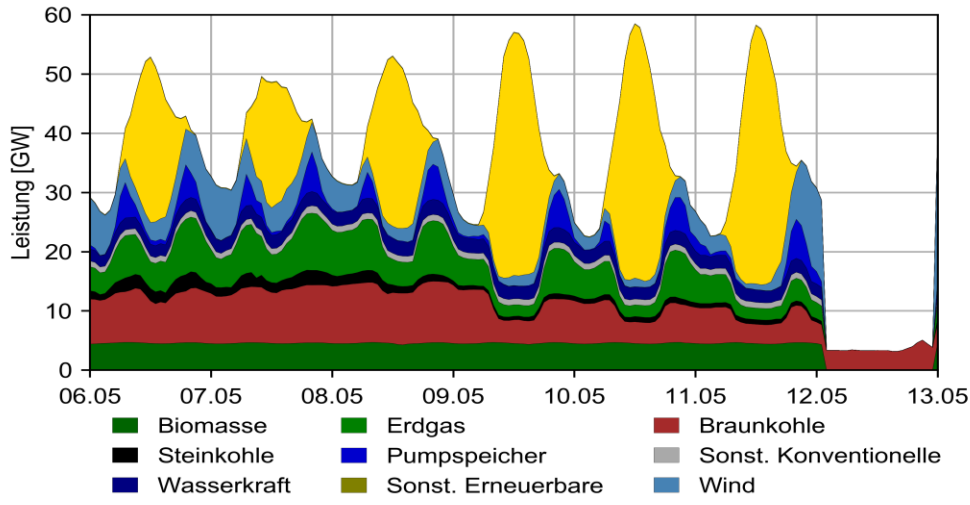
Kumulierte realisierte Erzeugung in Deutschland*
