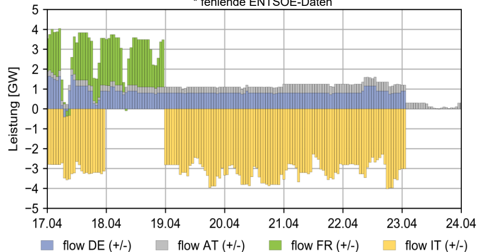
Netto kommerzielle Flüsse, kumuliert Import in CH (+) / Export aus CH (-) * fehlende ENTSOE-Daten
