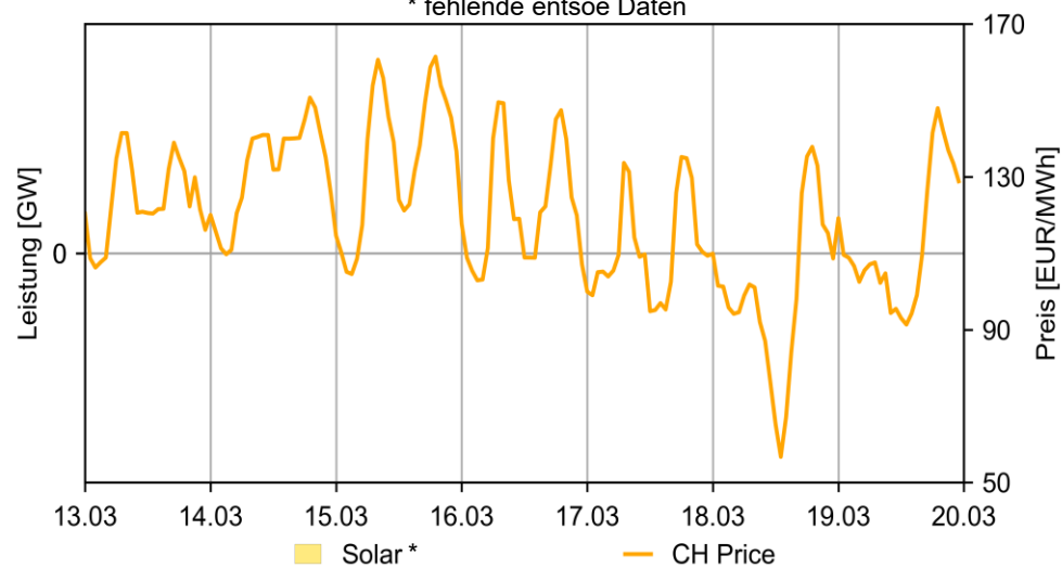
Realisierte kumulierte Erzeugung aus E.E und Day-Ahead Auktion Stundenpreis in der Schweiz * fehlende entsoe Daten
