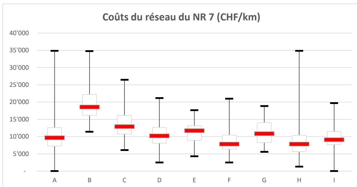
Diagramme en boîte des coûts du réseau du NR 7 (Quatre valeurs extrêmes ont été exclues).
