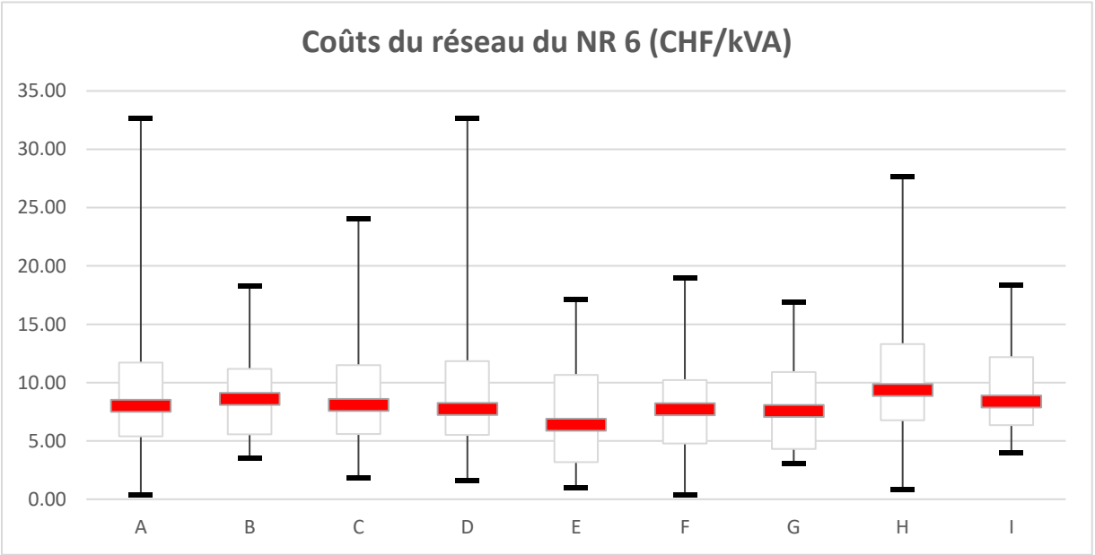
Diagramme en boîte des coûts du réseau du NR 6 (Deux valeurs extrêmes ont été exclues).
