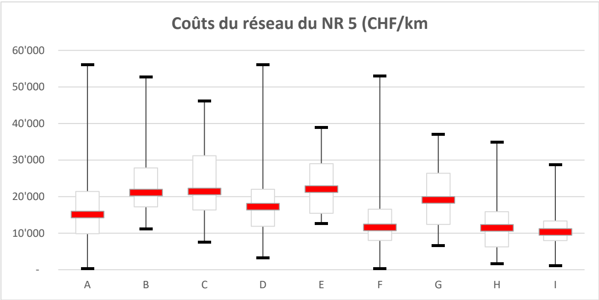
Diagramme en boîte des coûts du réseau du NR 5 (Une valeur extrême a été exclue).
