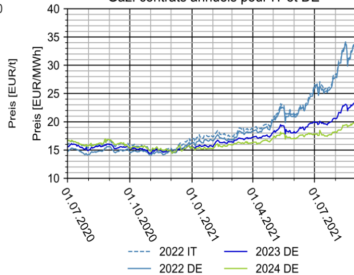
Gasjahreskontrakte für IT und DE Gaz: contrats annuels pour IT et DE
