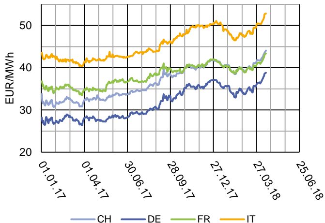
Strom Base Frontjahreskontrakte Électricité Base contrats annuels 2019
