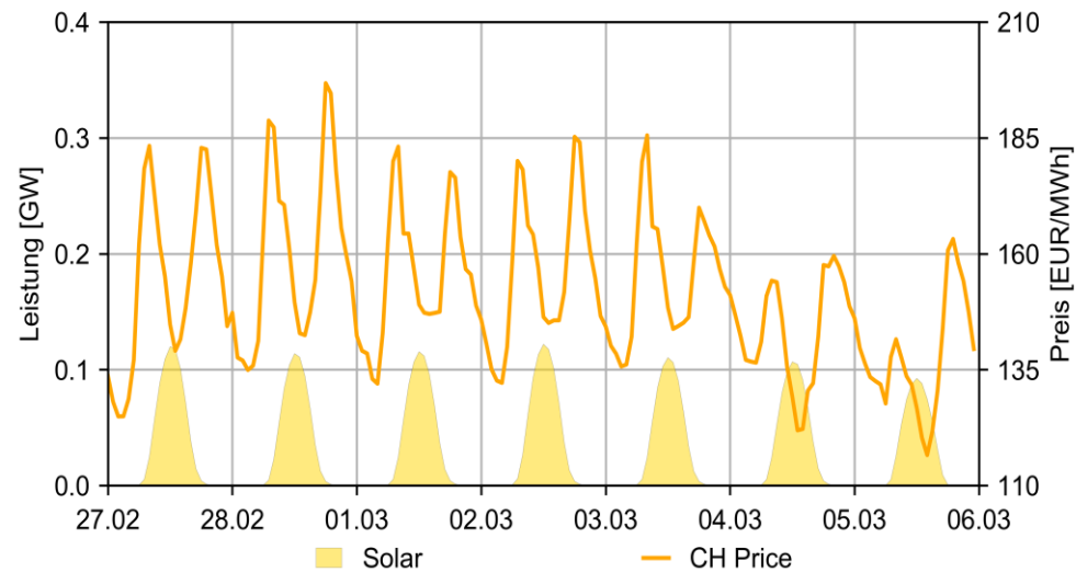
Prognostizierte kumulierte Erzeugung aus E.E. und Day-Ahead Auktion Stundenpreis in der Schweiz
