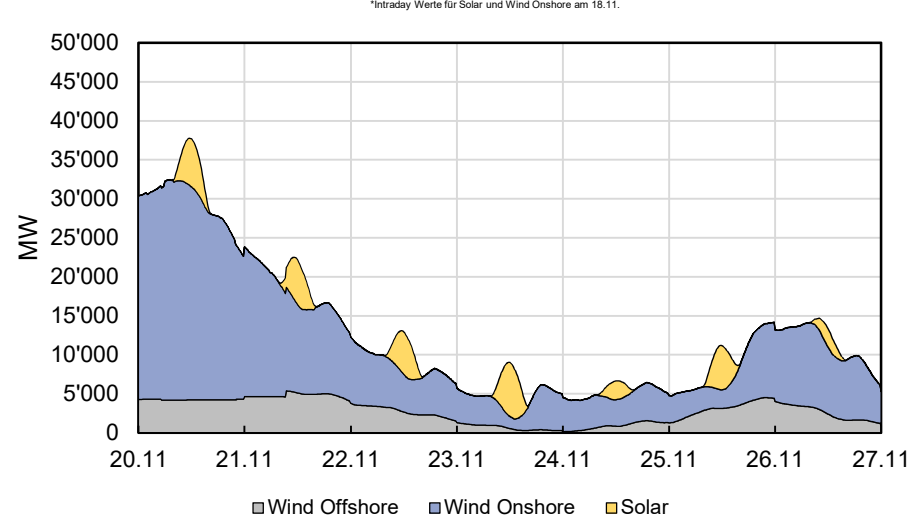
Kumulierte Erzeugung aus E.E. in DE: Prognose*
