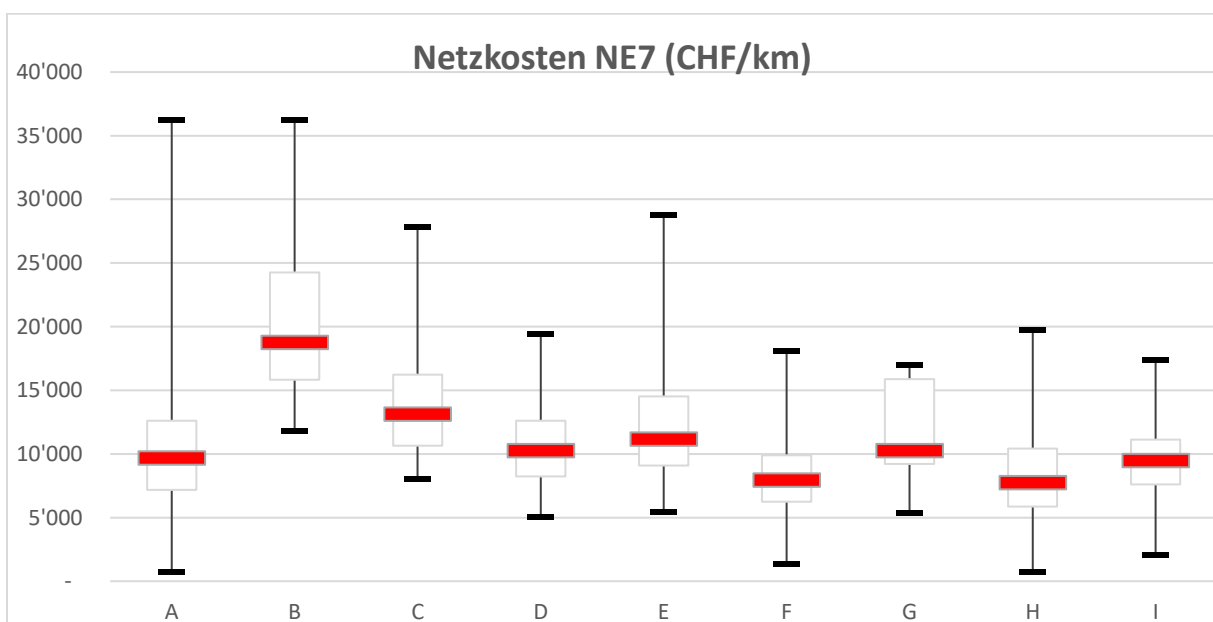
Boxplot Netzkosten Netzebene 7 (Drei Werte wurden aus der Darstellung ausgeschlossen)
