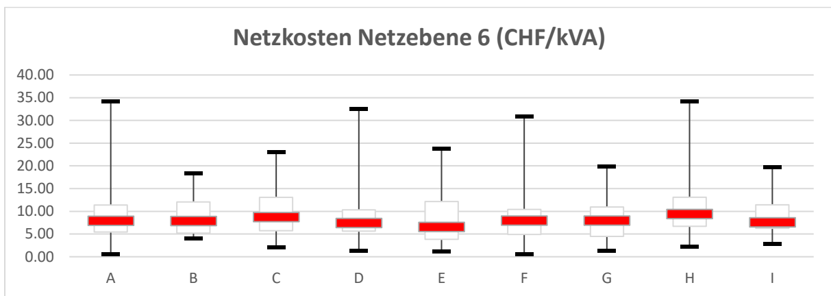
Boxplot Netzkosten Netzebene 6 (Zwei Werte wurden aus der Darstellung ausgeschlossen)
