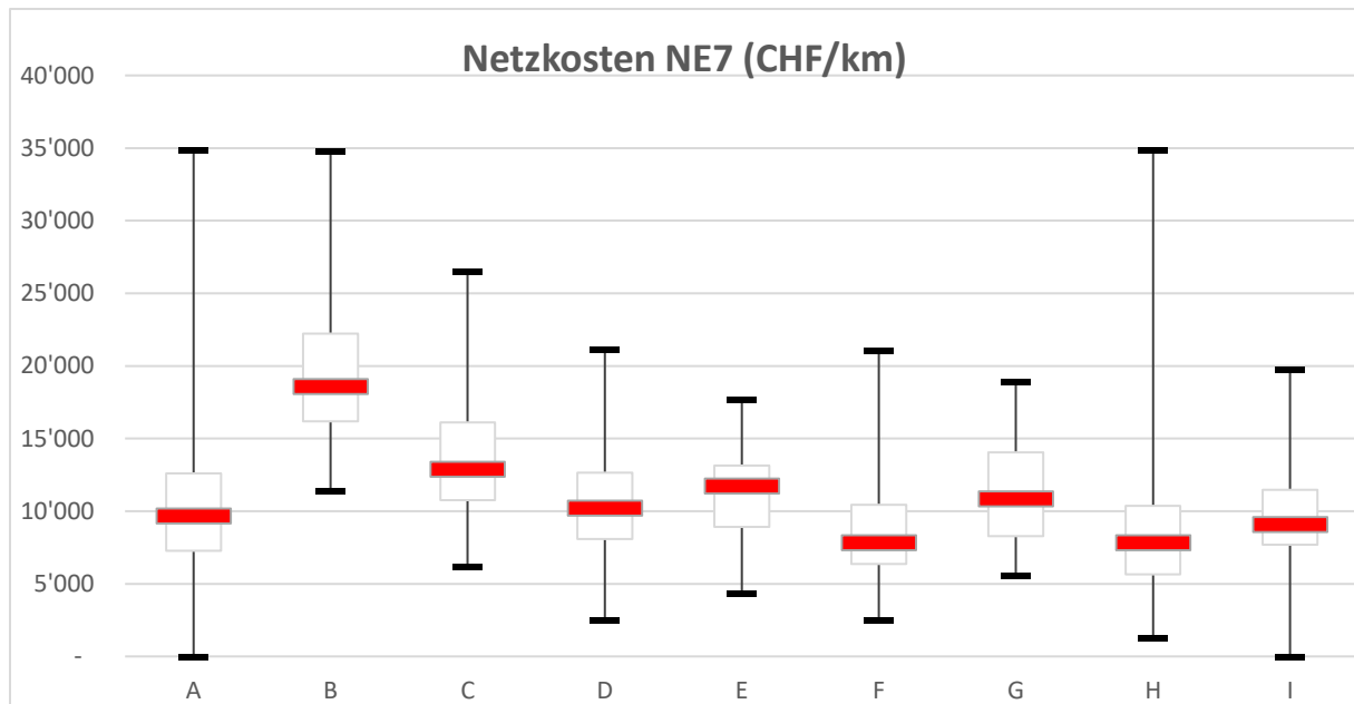
Boxplot Netzkosten Netzebene 7 (Vier Werte wurden aus der Darstellung ausgeschlossen)
