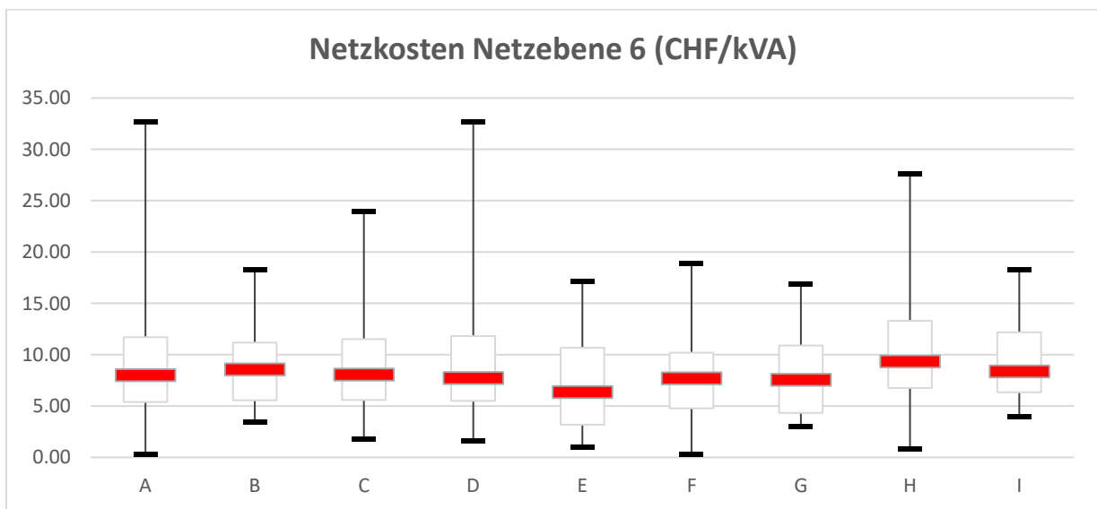
Boxplot Netzkosten Netzebene 6 (Zwei Werte wurden aus der Darstellung ausgeschlossen)
