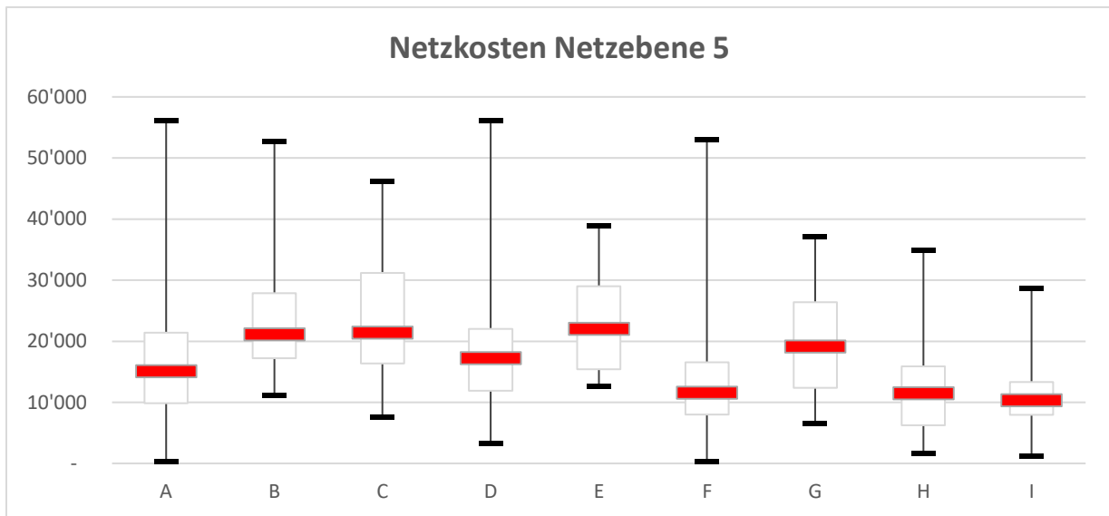
Boxplot Netzkosten Netzebene 5 (Ein Wert wurde aus der Darstellung ausgeschlossen)
