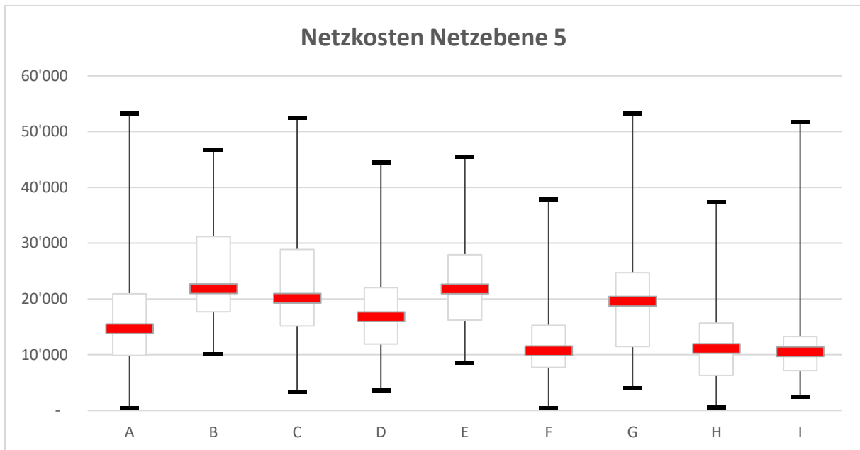
Boxplot Netzkosten Netzebene 5 (Ein Wert wurde aus der Darstellung ausgeschlossen)
