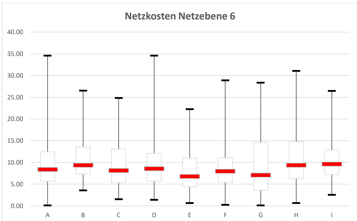
Boxplot Netzkosten Netzebene 6 (Fünf Werte wurden aus der Darstellung ausgeschlossen)
