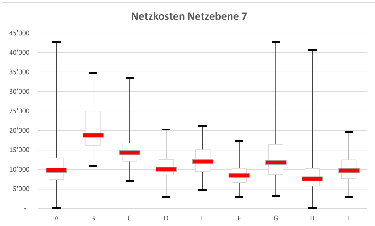
Boxplot Netzkosten Netzebene 7 (Drei Werte wurden aus der Darstellung ausgeschlossen)
